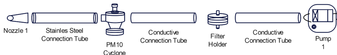
Figura 4. Rappresentazione schematica della linea 1
