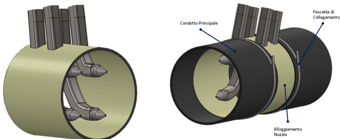
Figura 10. Sistema di Alloggiamento sonde (Nozzle)
