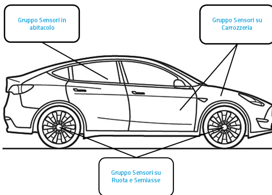
Figura 2. Schema indicativo delle modifiche da apportare al veicolo: Sensoristica VD
