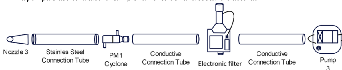
Figura 6. Rappresentazione schematica della linea 3
