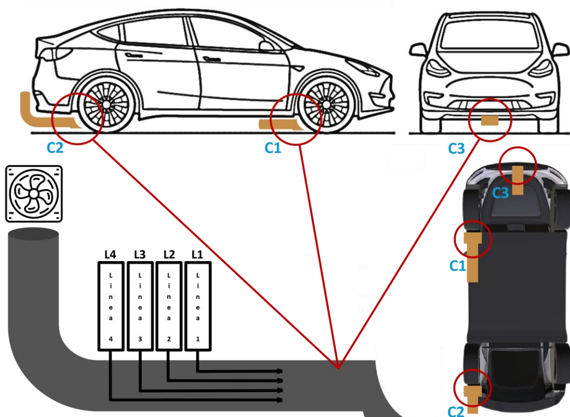
Figura 8. Illustrazione qualitativa e funzionale del posizionamento dei tre punti di campionamento posti sulla vettura
