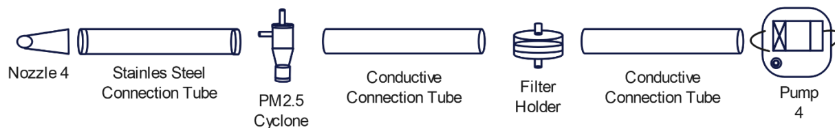
Figura 7. Rappresentazione schematica della linea 4
