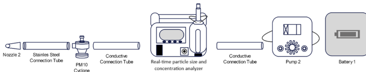
Figura 5. Rappresentazione schematica della linea 2
