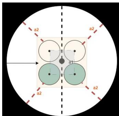
Figura 9. Disposizione Geometrica degli Ugelli (Nozzle) all'interno del tubo
