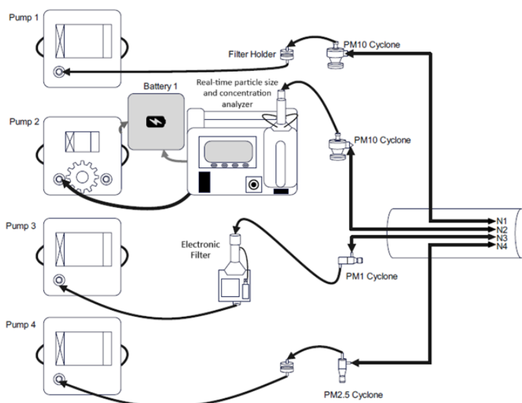
Figura 3. Configurazione finale della strumentazione di analisi e raccolta del particolato in base all'obiettivo del progetto
